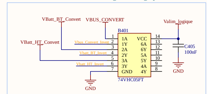
Inversion des signaux logiques
