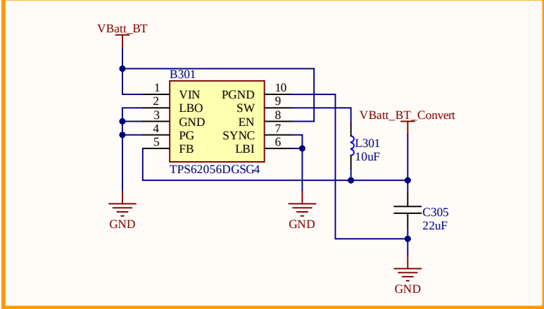
Conversion de la tension BT en 3,3 V
