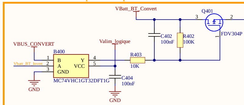
Ordre de priorité 2 pour l'alimentation HT
