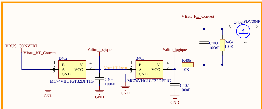
Ordre de priorité 2 pour l'alimentation HT
